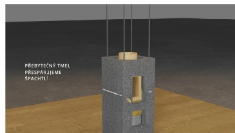
09. Přespárování přebytečného tmelu
