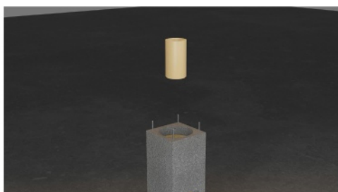
19. Osazení rovné keramické vložky
