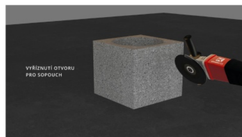
15. Výřez otvoru pro sopouch
