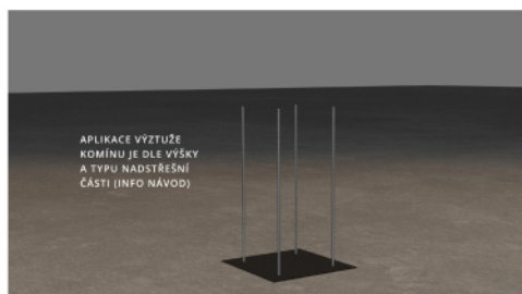
01. Výztuž komína
