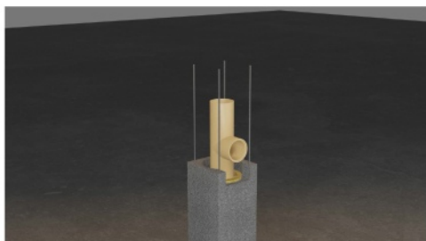
16. Osazení sopouchu
