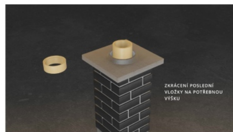
24. Zkrácení poslední vložky
