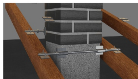
27. Kotvení komína do krovu
