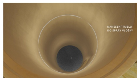
12. Nanesení tmelu do spoje vložky
