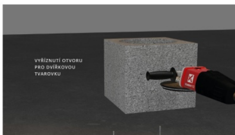
08. Výřez další tvárnice pro dvířka
