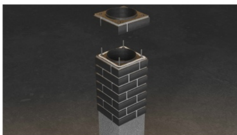
22. Zakončovací prstenec
