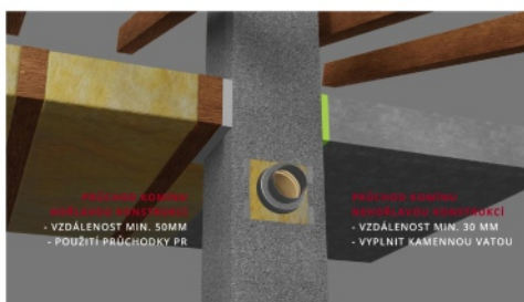
29. Bezpečný prostup konstrukcí
