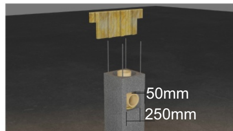
18. Izolace nad sopouchem
