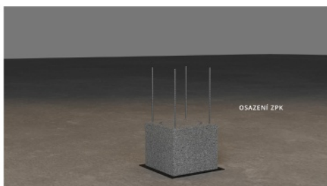
02. Založení první tvárnice
